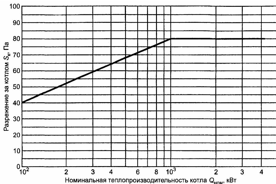
Рисунок 2 — Максимальное разрежение за котлом на естественной тяге
