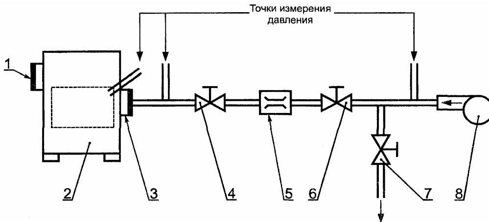
1 — патрубок уходящих газов; 2 — испытуемый котел; 3 — амбразура горелки; 4 — регулирующий орган 1; 5 — измеритель расхода; 6 — регулирующий орган 2; 7 — регулирующий орган 3; 8 — вентилятор
